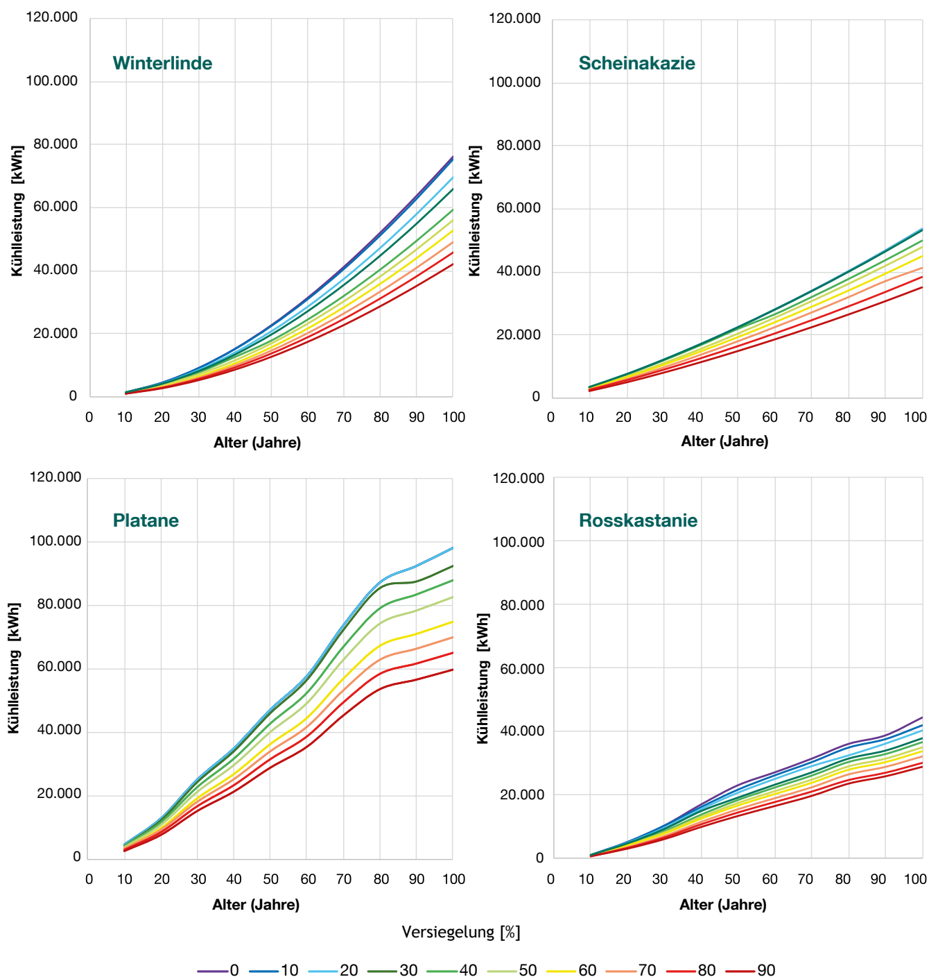
Abbildung 20: Kühlung durch Transpiration von Winterlinden, Scheinakazien, Roskastanien und Platanen in Bayern mit steigendem Alter und bei verschiedenen Versiegelungsgraden für das gegenwärtige Klima.
