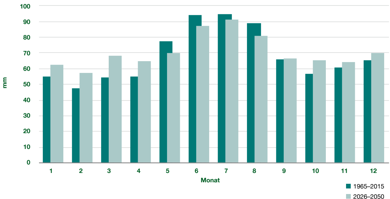
Abbildung 8: Mittlere monatliche Niederschlagssummen für das aktuelle Klima (1965–2015) und für die nahe Zukunft (2026–2050) des Szenario A1B im Mittel der sechs bayerischen Städte.
